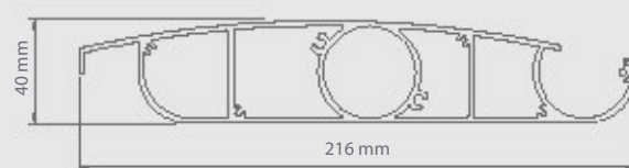
Prierez lamelou
