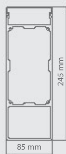
Prierez nosníkom
