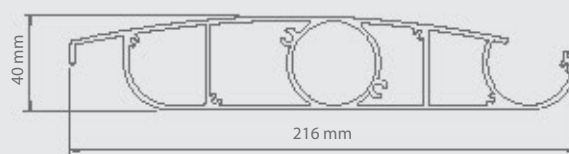
Prierez nosníkom
